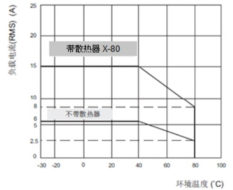
最大负载电流与环境温度曲线(15A)
