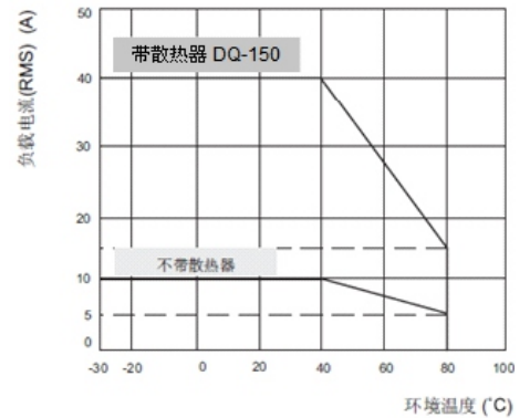
最大负载电流与环境温度曲线(40A)
